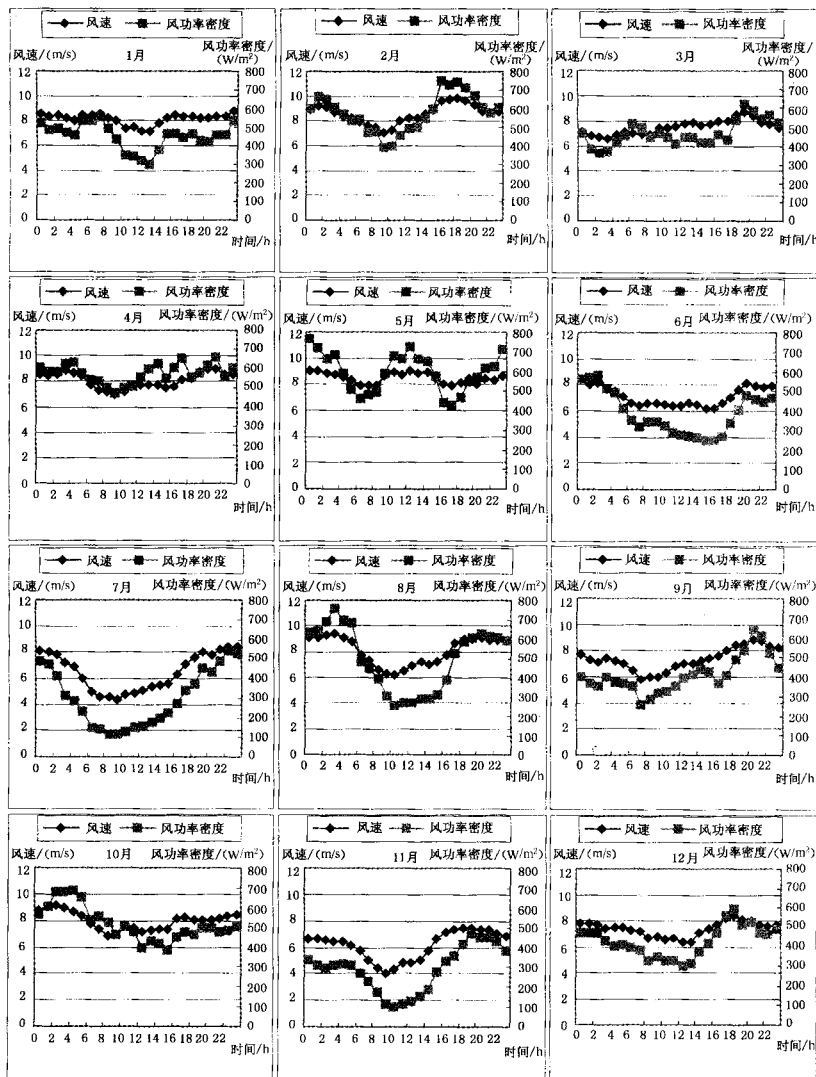
图 D6 各月的风速和风功率密度日变化曲线图
