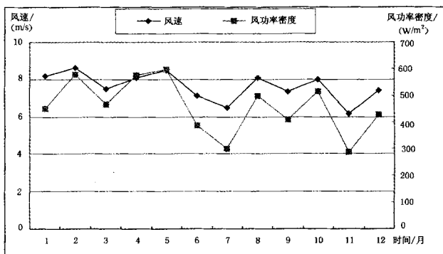
图 D2 风速和风功率密度年变化曲线图
