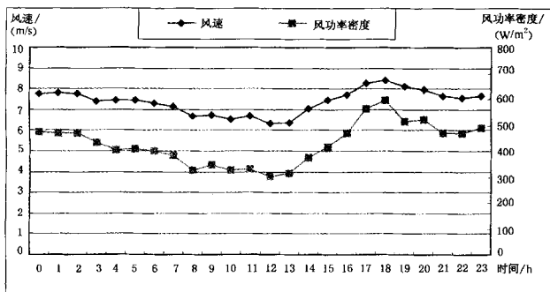
图 D1 全年的风速和风功率密度日变化曲线图
