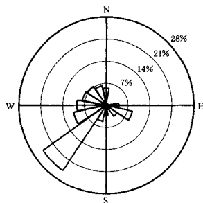
图 D5 全年的风能玫瑰图
