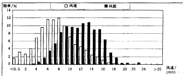
图 D3 全年的风速和风能频率分布直方图
