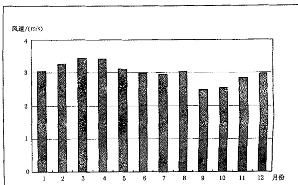
图 D9 与风场测风塔同期的相关长期测站风速年变化直方图
